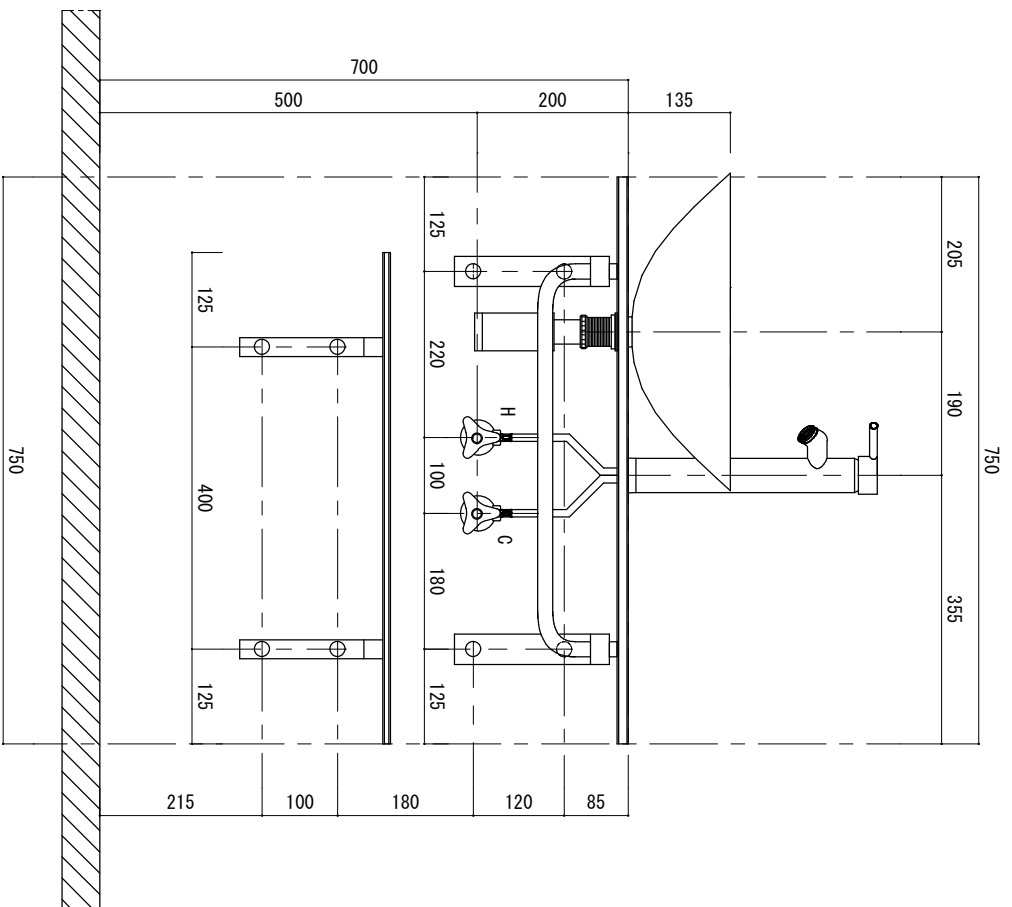
立面図
