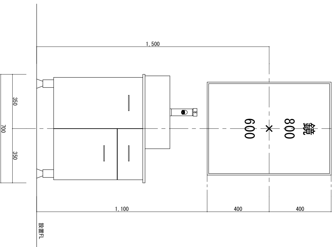
鏡取り付け図
