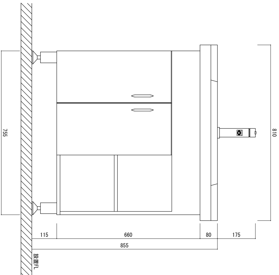
正面図
